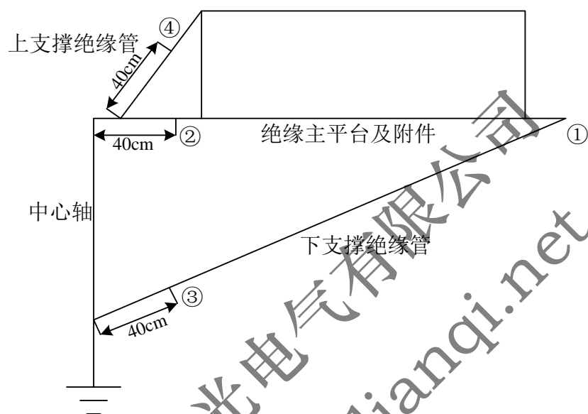
图B.4 绝缘平台电气试验布置图 绝缘手套交直流耐压试验接线图见图B.5。
