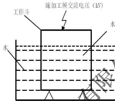
图B.14c) 绝缘斗层向耐压试验
