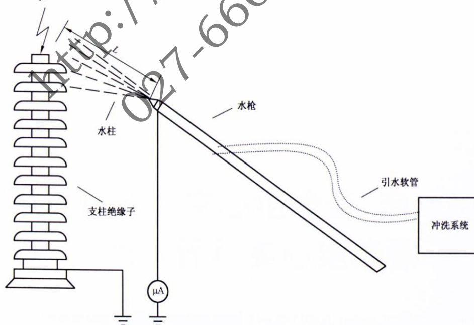
图B.15 水冲洗工具泄露电流试验布置图
