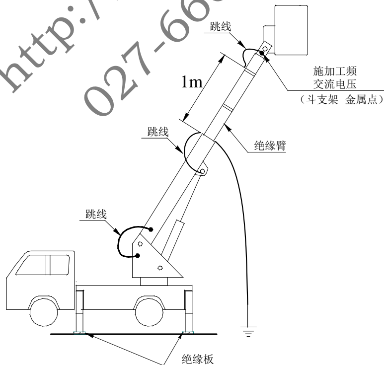
图 B.14d) 绝缘外斗表面交流耐压和泄漏电流试验
