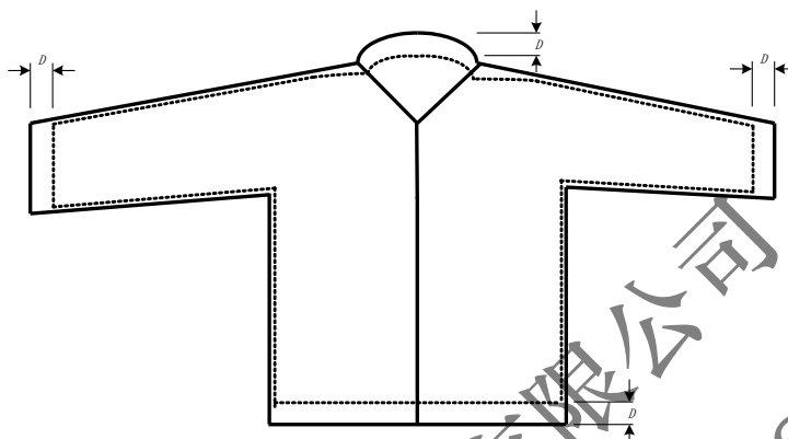
图 B.7b) 绝缘上衣内电极布置示意图
