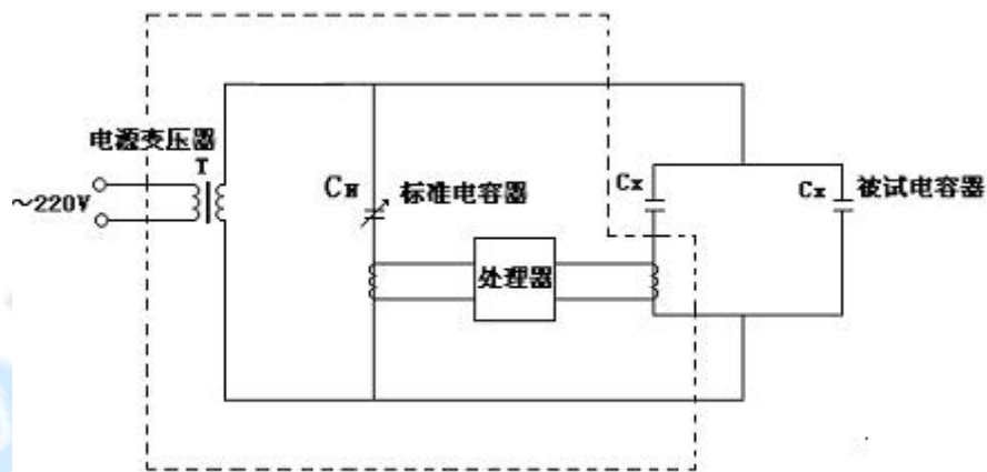
图1 工作原理
