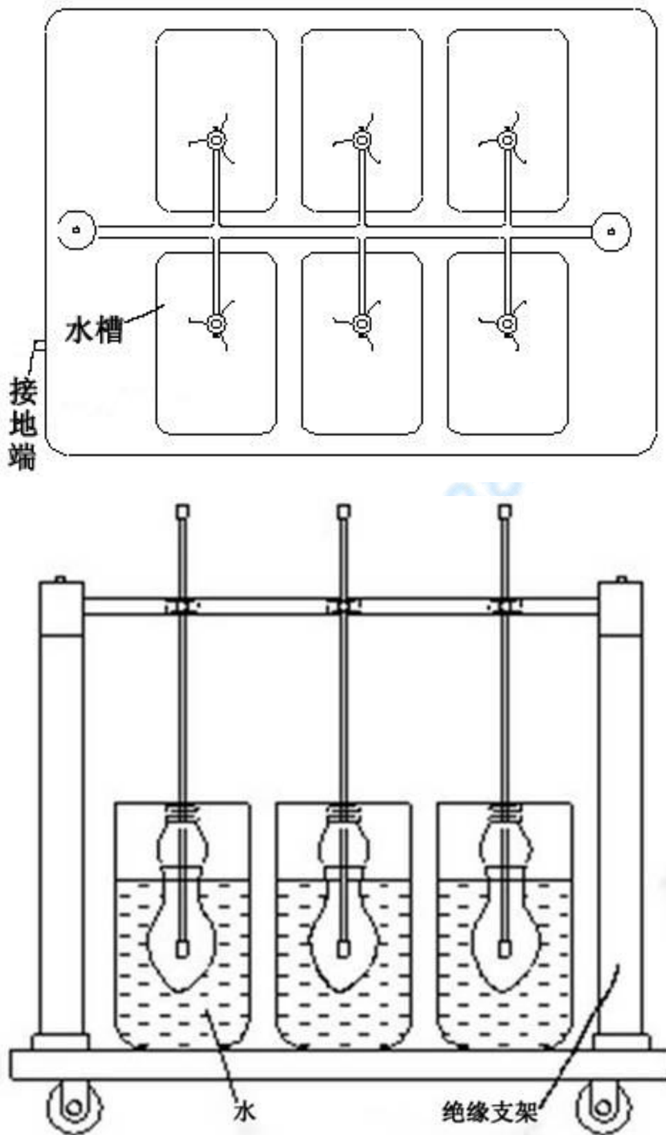
图 3-2 绝缘靴（手套）试验台
