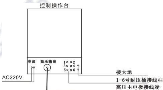
图 1 接线示意图
