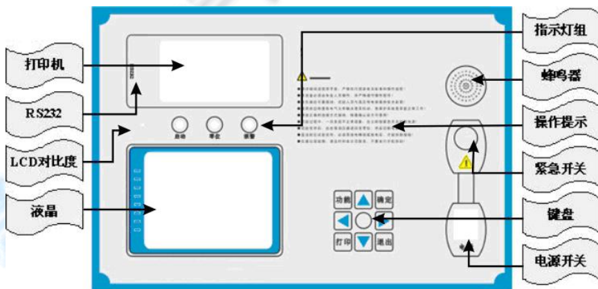
图 2 面板结构图
