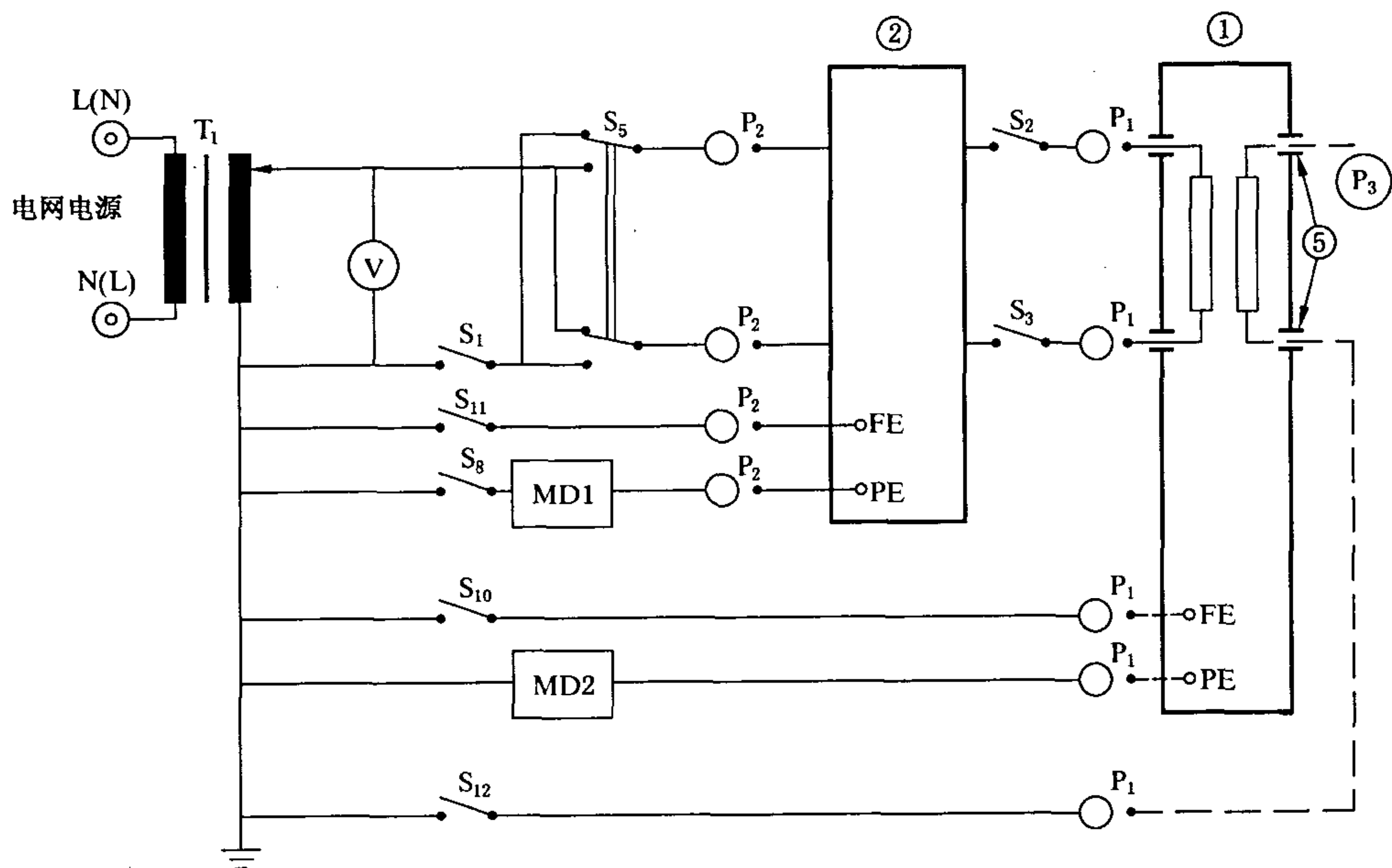
图 16 具有或没有应用部分的 I 类设备对地漏电流的测量电路[19.4 f)和表 4 的注] 用图 10 的测量供电电路的图例
