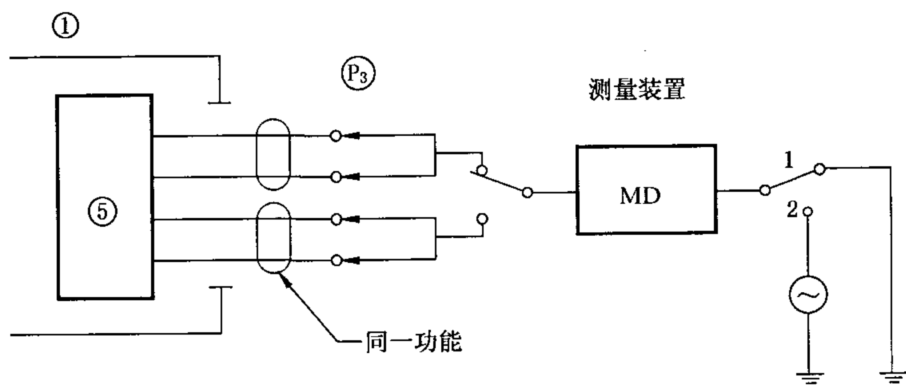
带 BF 型应用部分的设备 轮流地从应用部分的同一功能连在一起的所有患者连接线测 图中的符号说明见图 27 后的说明。
