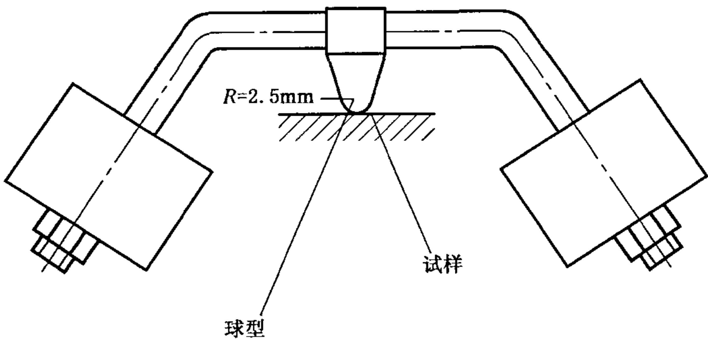
图 48 球压试验装置(见 59.2)
