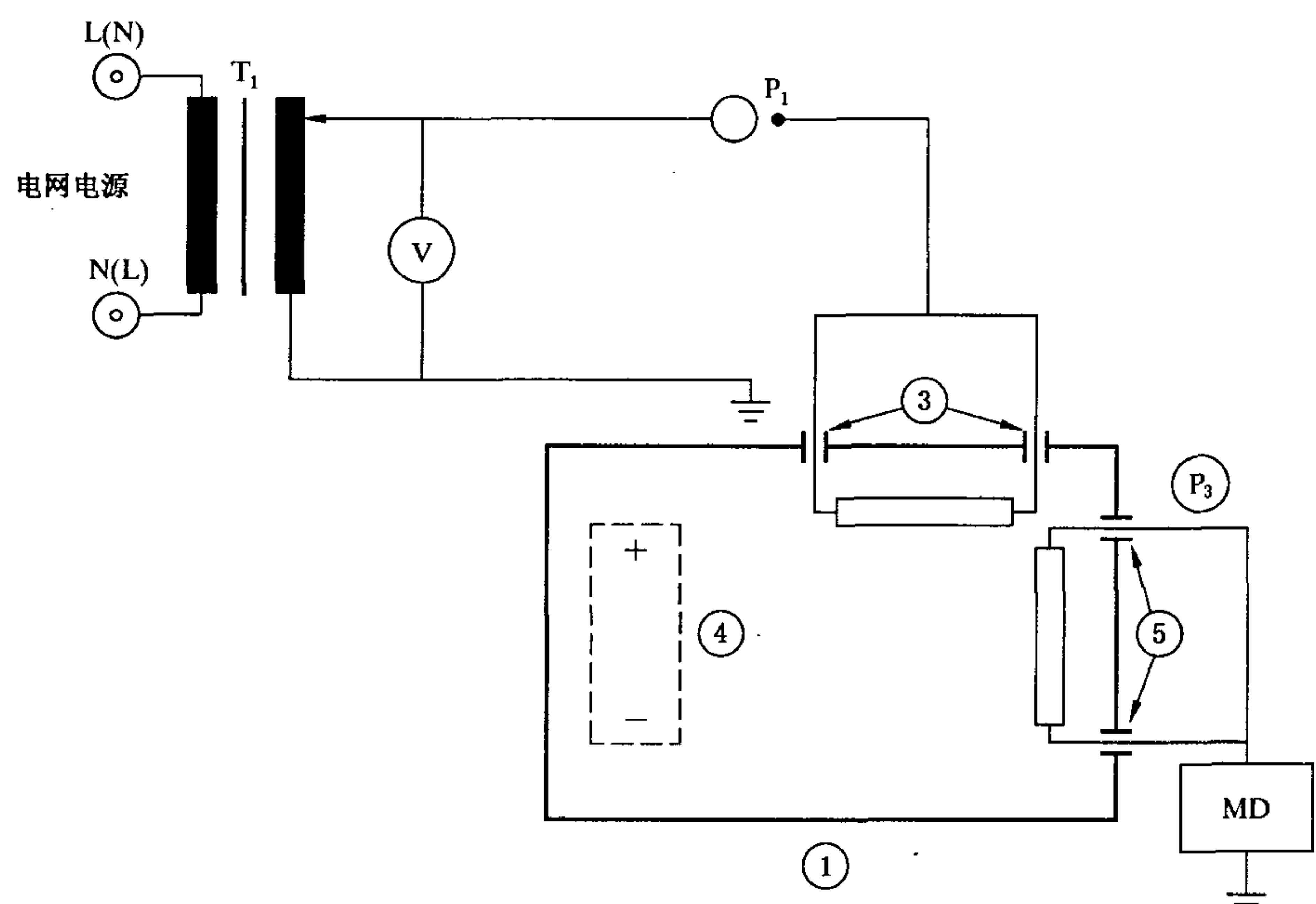
图 25 内部电源设备,由信号输入部分或信号输出部分上的外来电压引起的从应用部分至地的患者漏电流的测量电路[见 19.4 h)]
