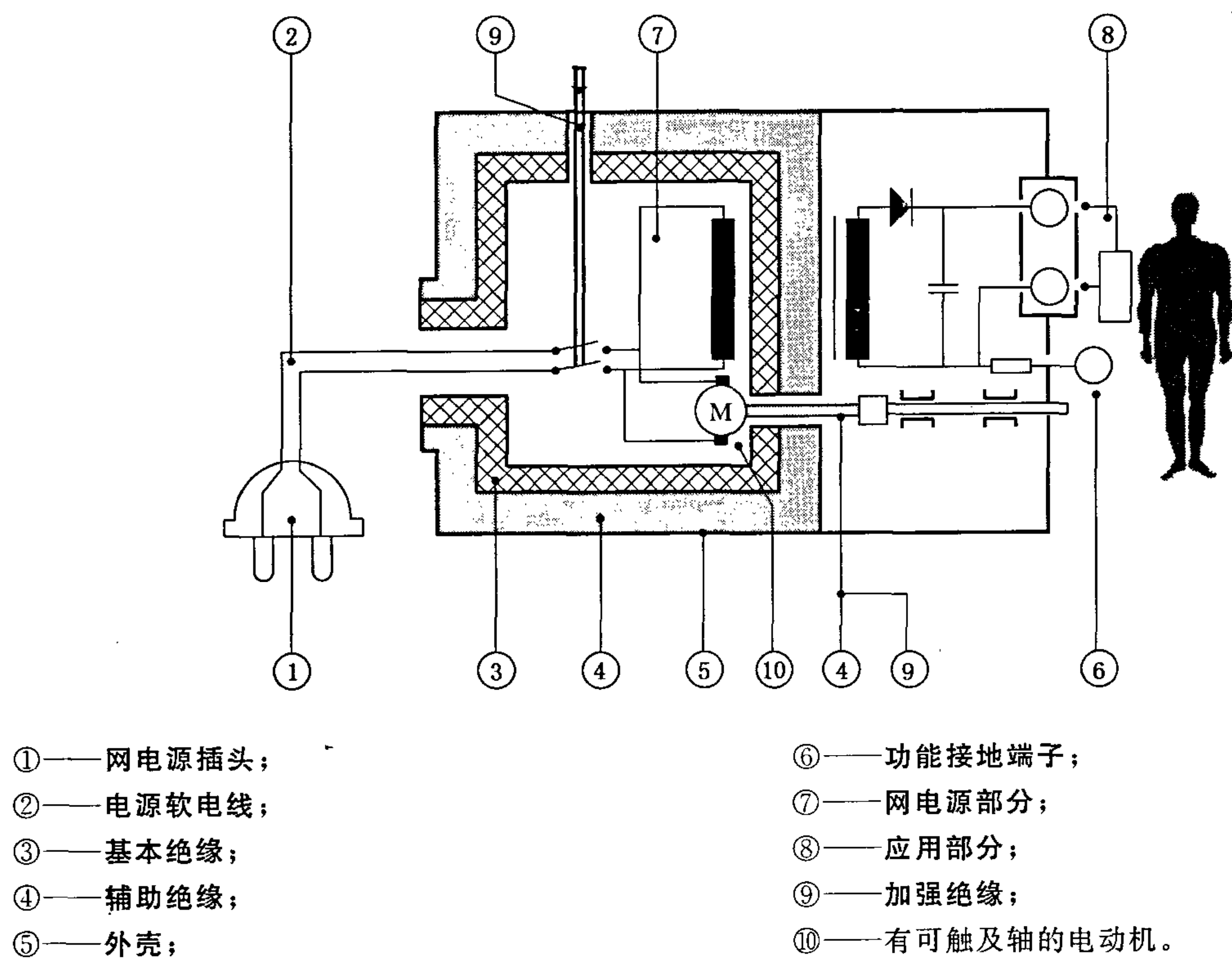
图 3 带金属外壳 II 类设备的图例(见 2.2.5)
