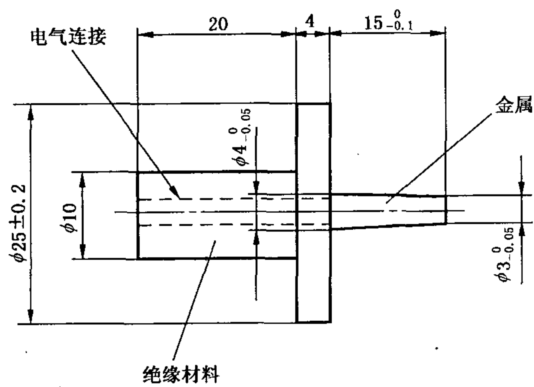
图 8 试验针(见第 16 章)
