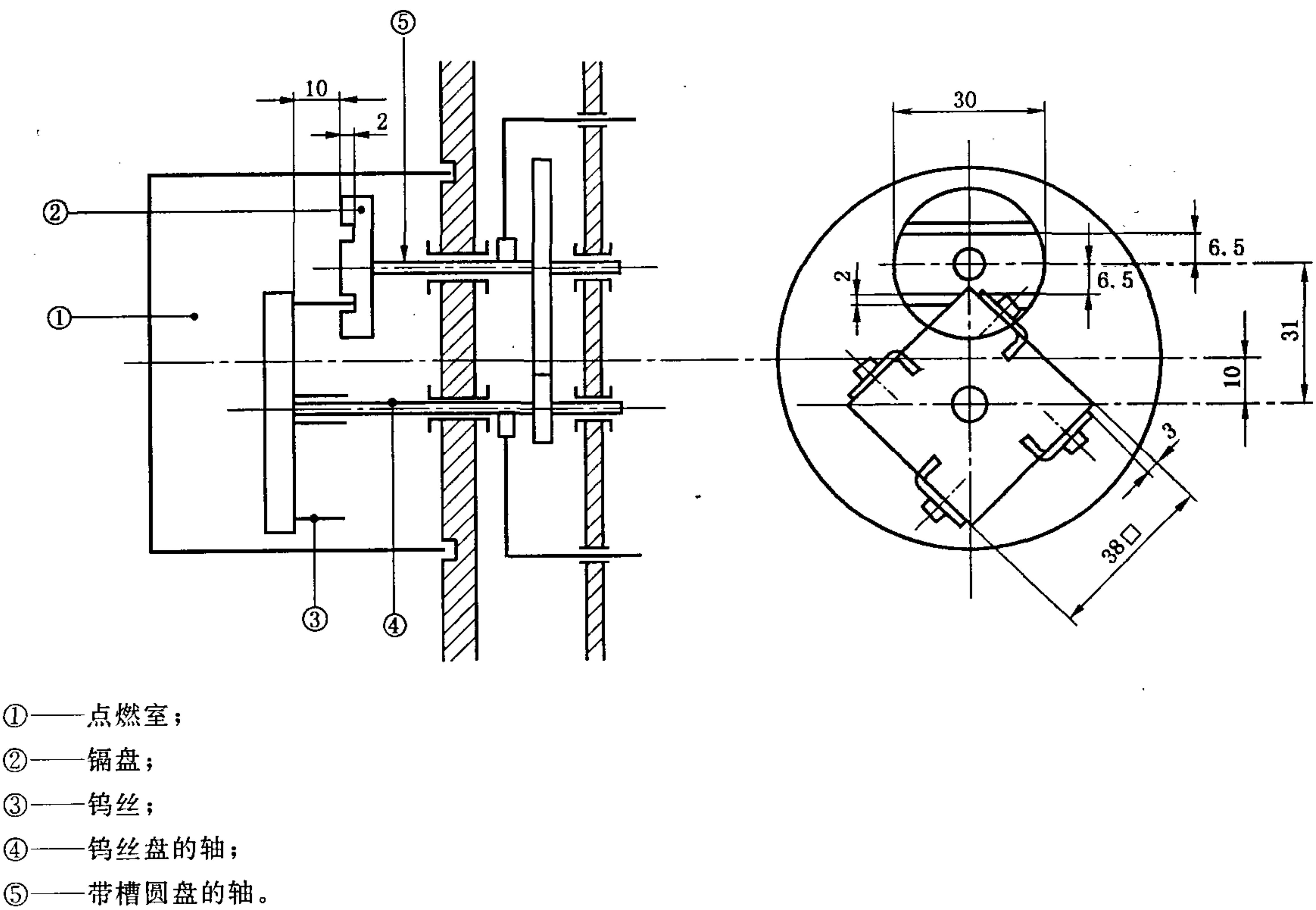
图 F.1 试验装置
