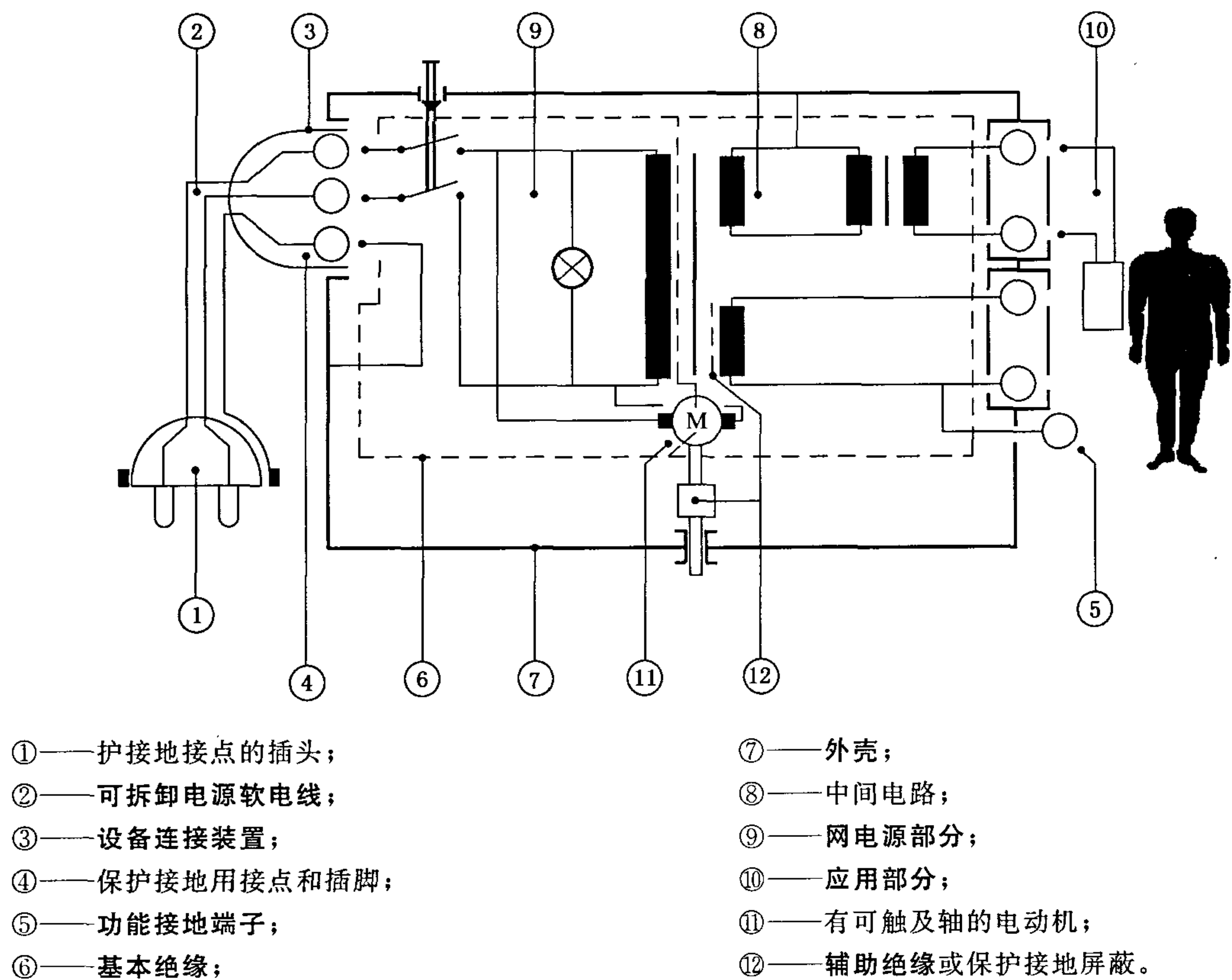
图 2 I 类设备的图例(见 2.2.4)
