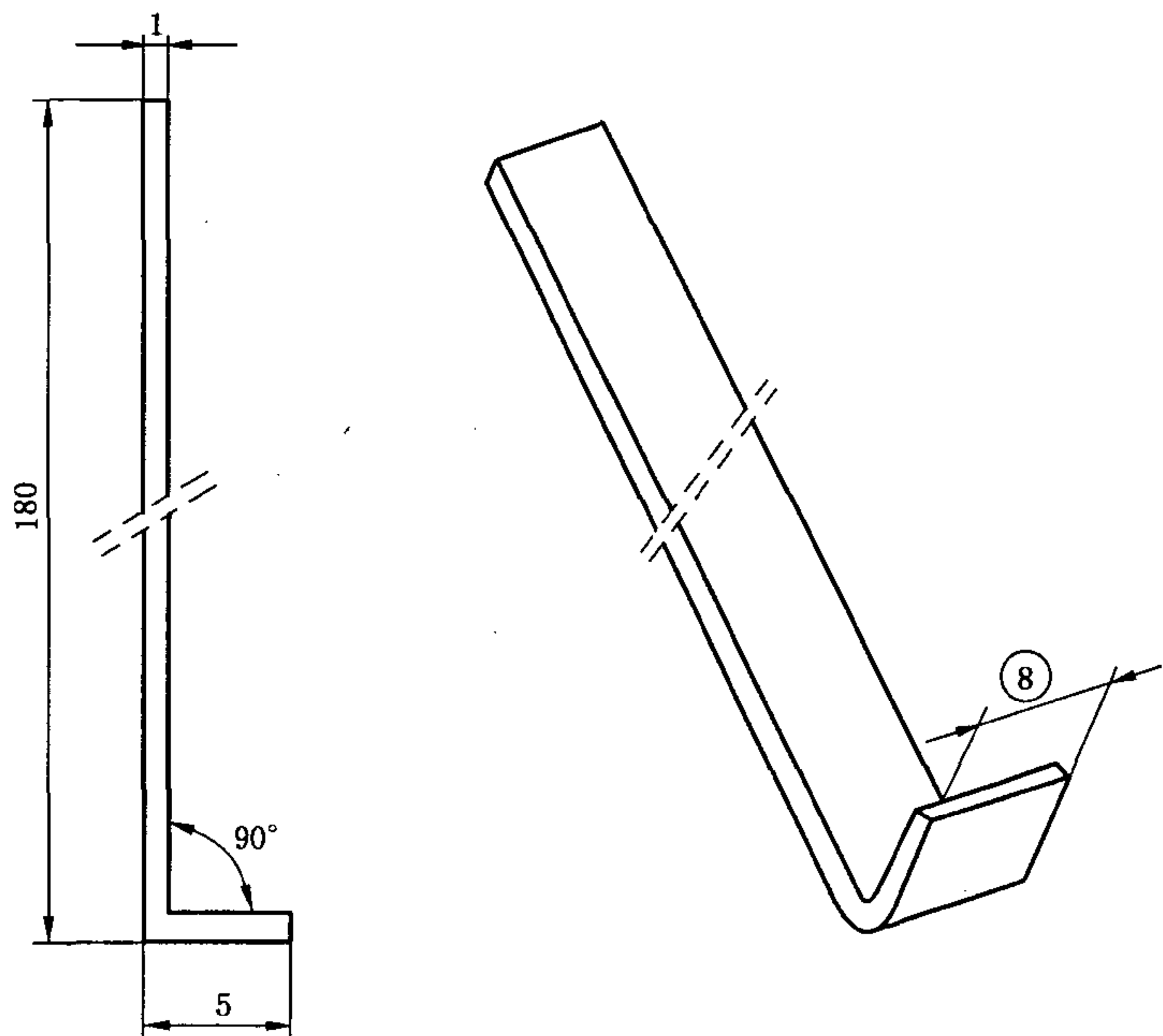
图 9 试验钩(见第 16 章)
