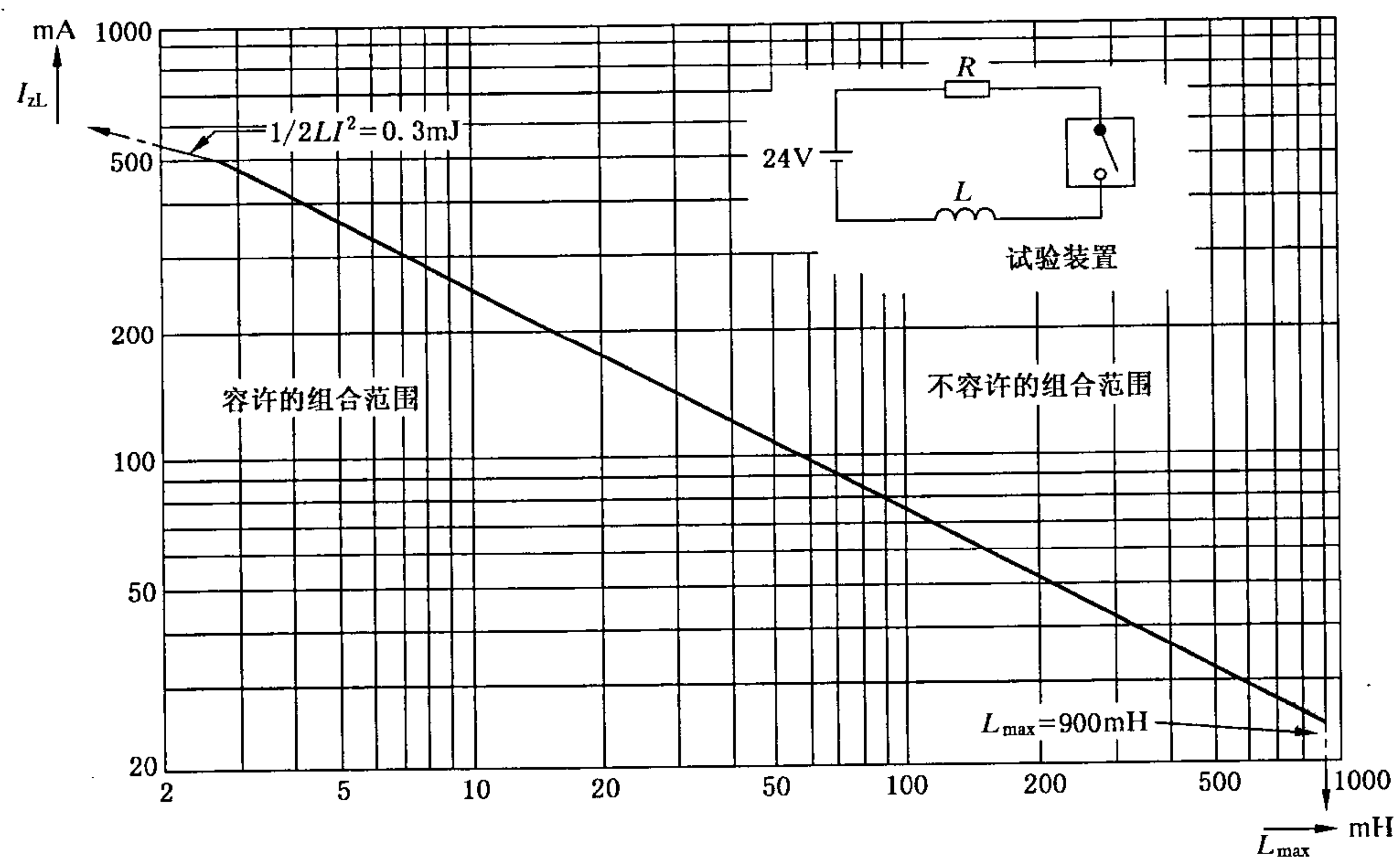
图 31 在乙醚蒸气和空气混合成的最易燃气体中电感电路上测得的最大容许电流 I_{zL} 和电感 L_{\max} 的函数关系(见 40.3)
