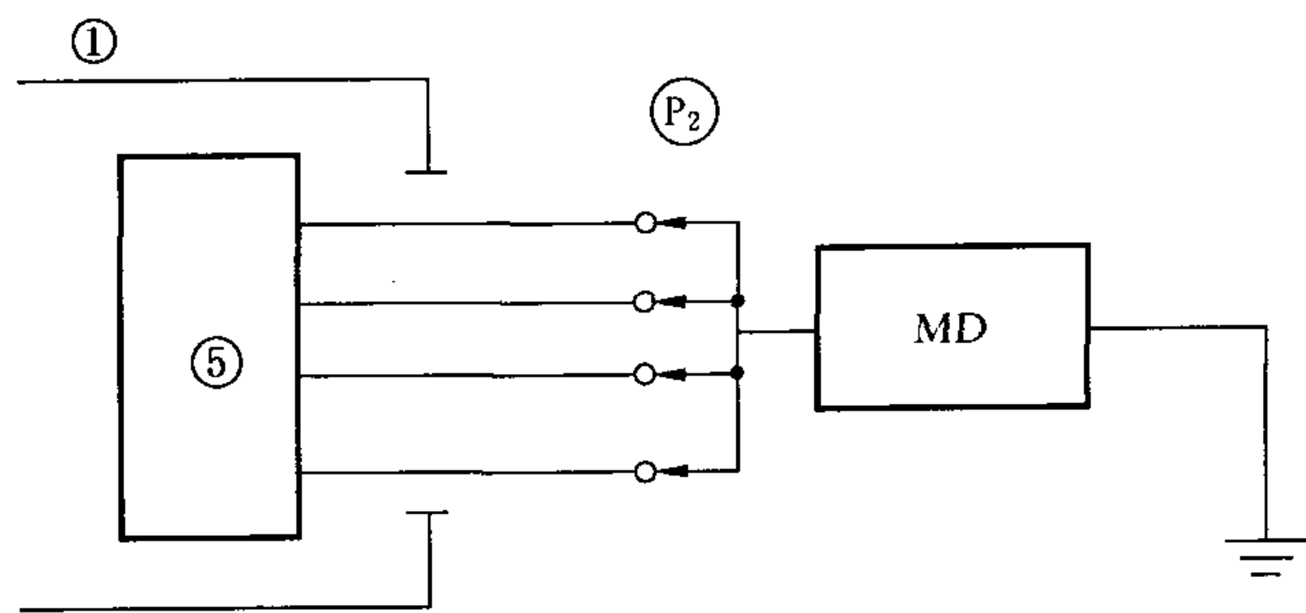
带 B 型应用部分的设备 从连在一起的所有患者连接线测 图中的符号说明见图 27 后的说明。
