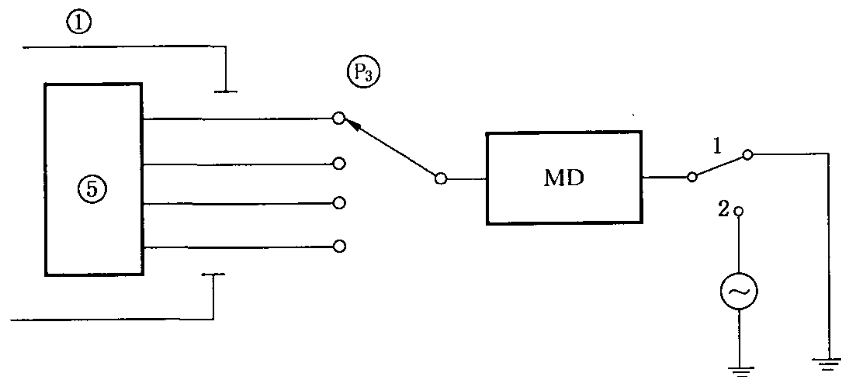
带 CF 型应用部分的设备 轮流地从每一患者连接线测 图中的符号说明见图 27 后的说明。 测量患者辅助电流时应用部分连接的示例(说明见图 27 后的说明)
