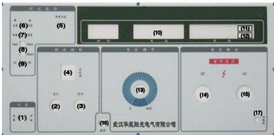
图（2）数显式耐压测试仪前面板示意图
