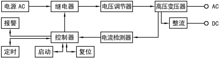
图 (1): 全数显耐压仪工作原理方框图
