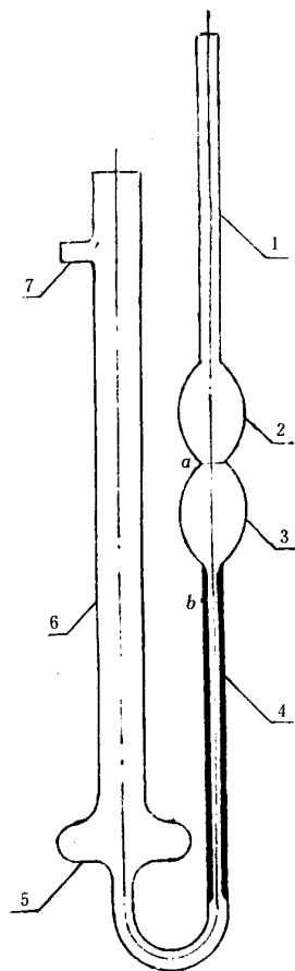
毛细管粘度计图
