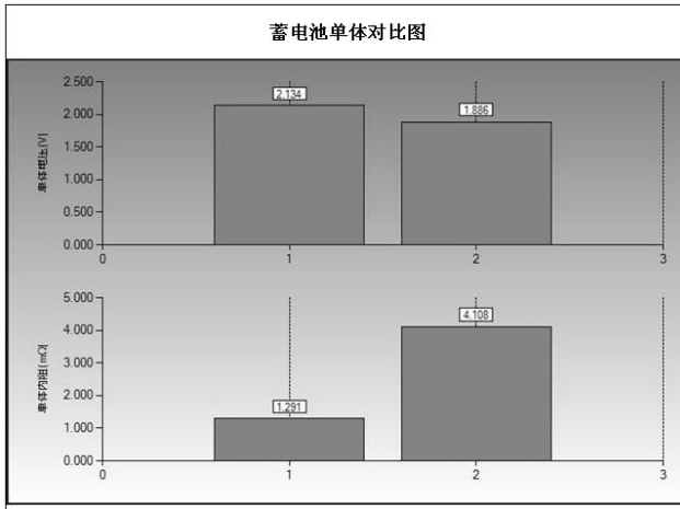
图 4.5-3 单体对比图
