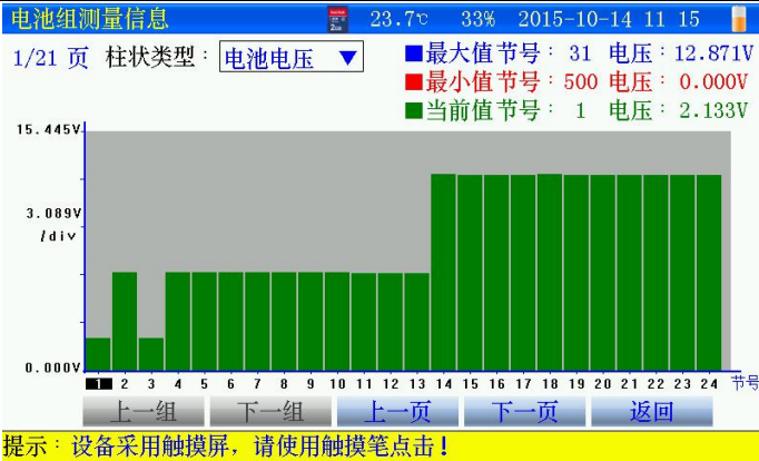
图 3.5.4-1 电池组柱状图界面
