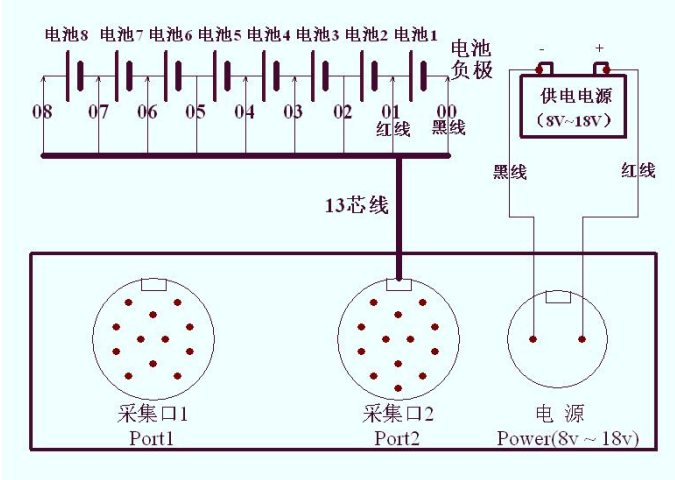
图 2.4.4-1 8 节 6V 电池与 1 个单体模块连接图
