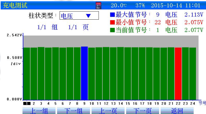
图 3.3.4-1 单体电压柱状图
