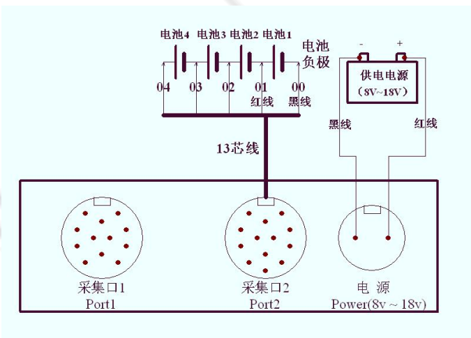
图 2.4.4-2 4 节 12V 电池与 1 个单体模块连接图
