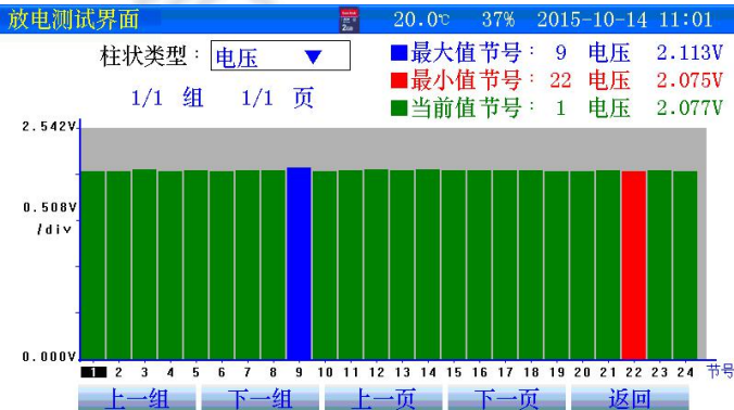
图 3.2.4-1 单体电压柱状图
