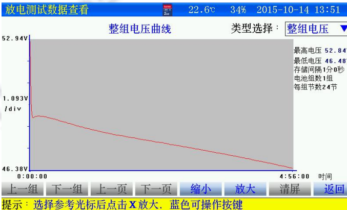
图 3.7.4 整组电压曲线界面
