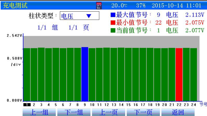
图 3.3.4-1 单体电压柱状图
