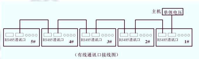
图 2.4.4.4 有线通讯口接口图
