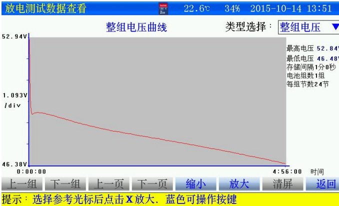
图 3.5.4 整组电压曲线界面
