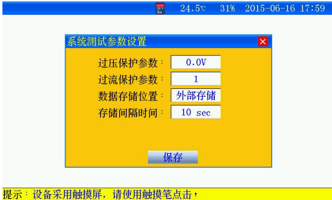
图 3.10 数据存储时间设置界面
