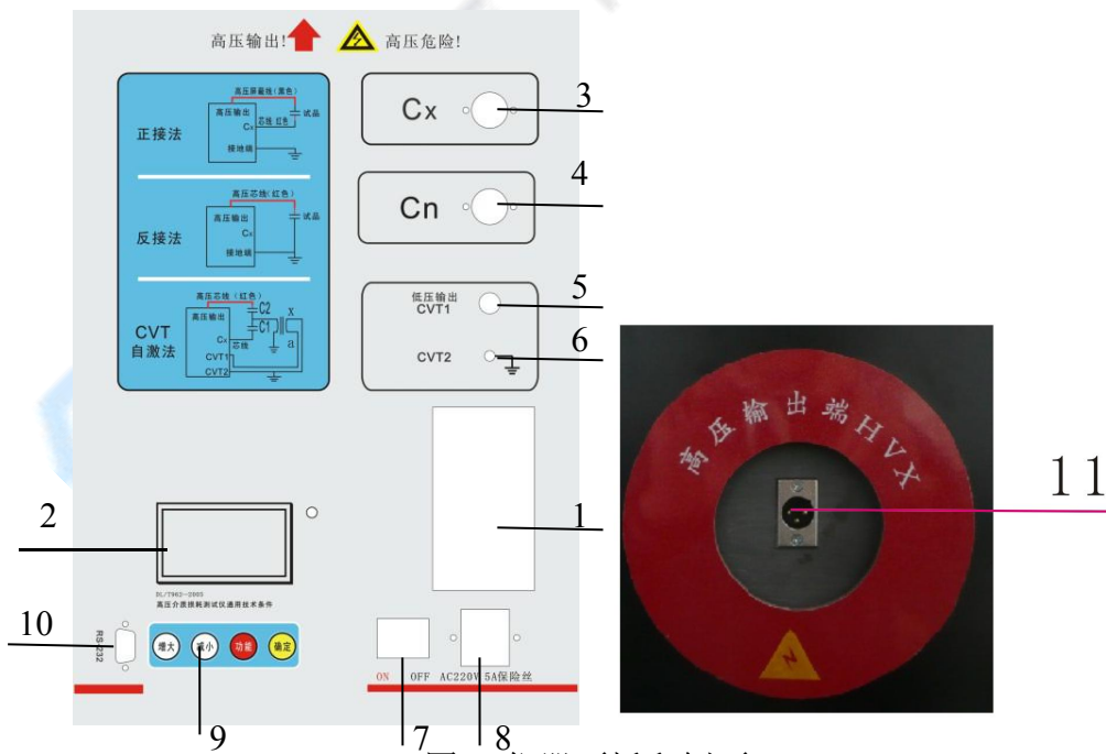
图 1 仪器面板和侧面
