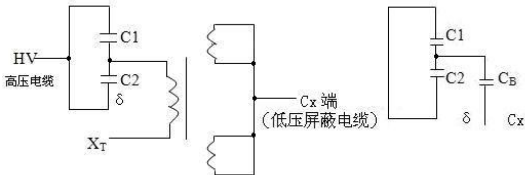
图 12 中压互感器（正接线）
