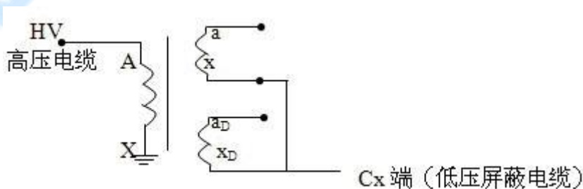
图 9 末端屏蔽法接线
