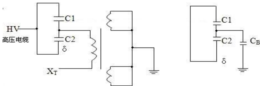
图 11 中压互感器（反接线）
