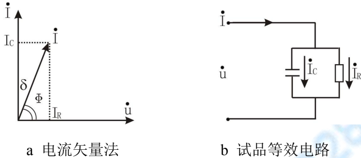
图 4 试品等效电路
