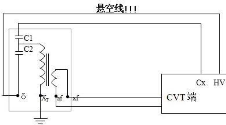
图 13 电容 C1 和 \text{tg } \delta 1 , C2 和 \text{tg } \delta 2 的接线
