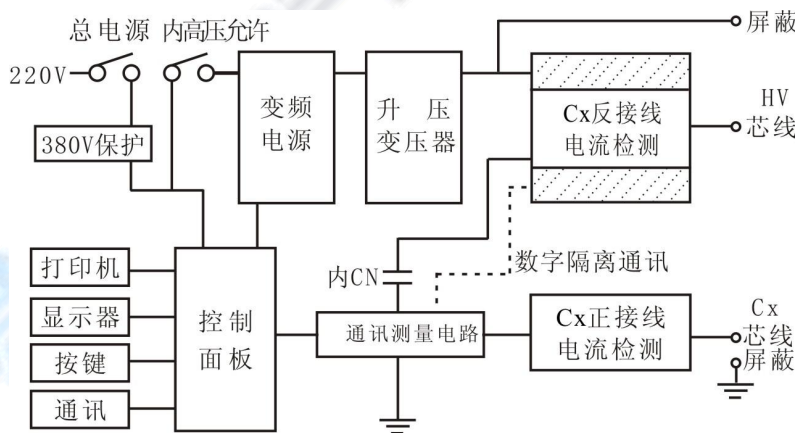
图 2 仪器结构图
