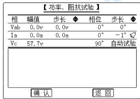
功率阻抗
