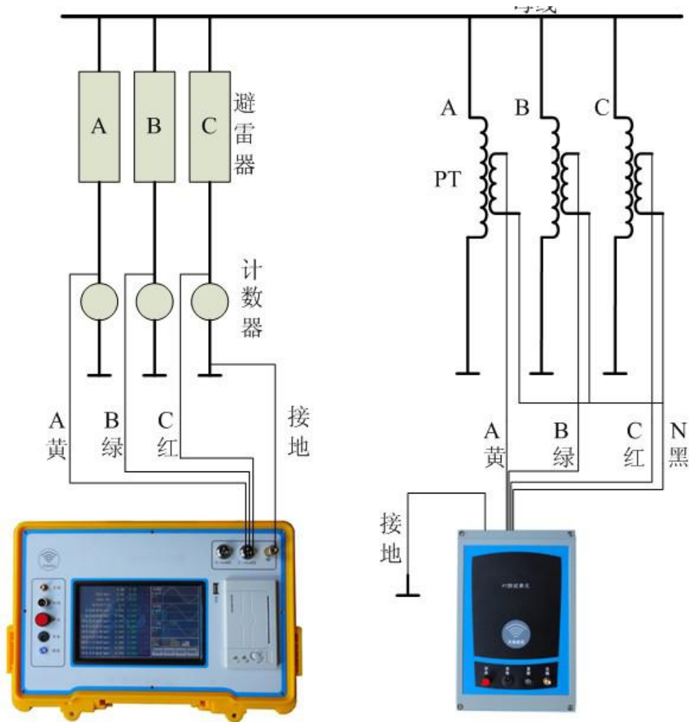
图 3 测试线接线示意图
