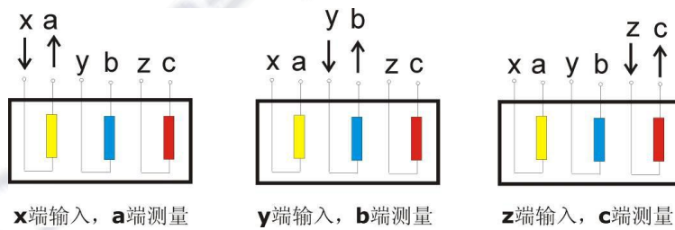
图6 外连接△接线
